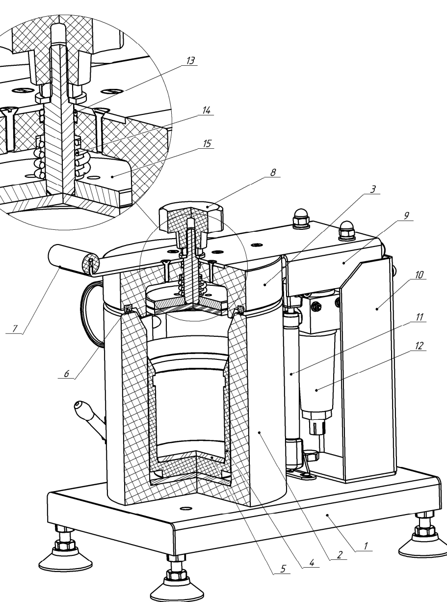
Рисунок 1. Машина укупорочная («Твист-Офф») ИПКС-127В, ИПКС-127-01В, ИПКС-127В/5ст
