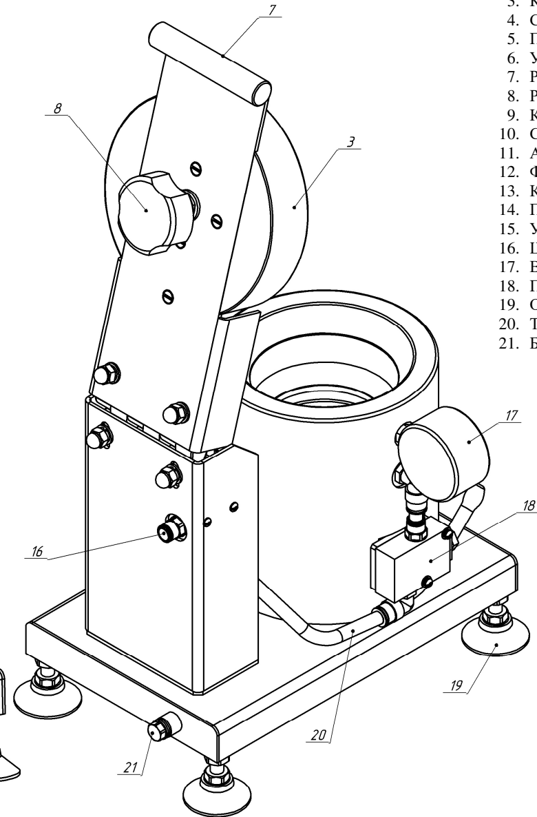
Рисунок 1. Машина укупорочная («Твист-Офф») ИПКС-127В, ИПКС-127-01В, ИПКС-127В/5ст
