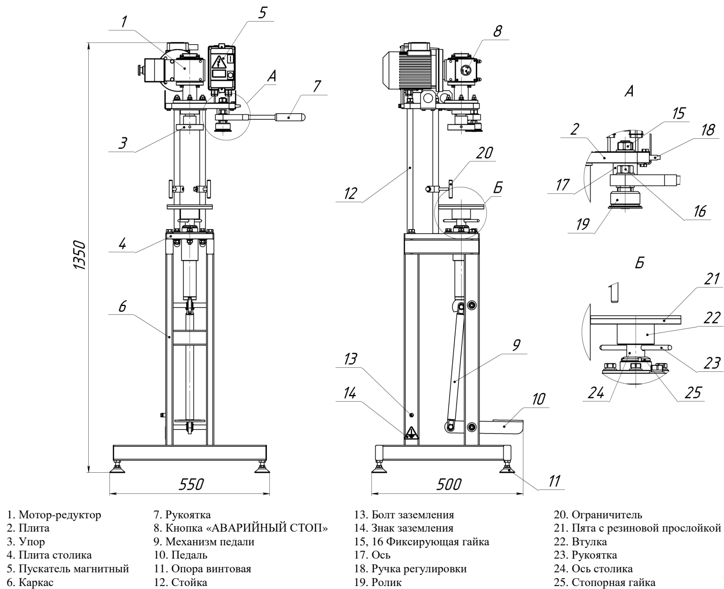
Рисунок 2. Машина укупорочная (закатка жестяных и стеклянных банок) ИПКС-127УЗ в комплектации для закатки стеклянных банок
