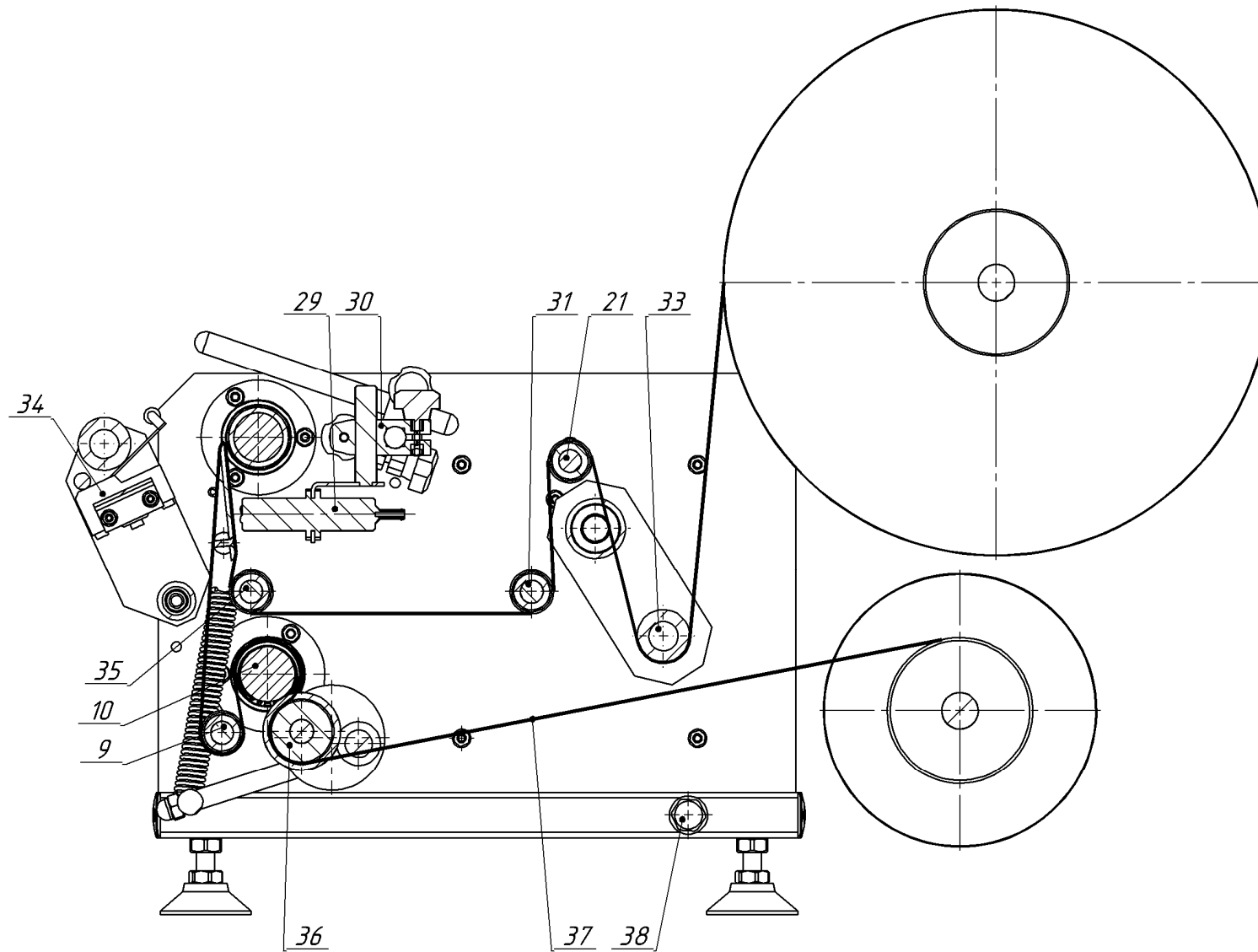
Рисунок 1, 6. Установка нанесения этикеток ИПКС-099Ц. Схема протяжки ленты.
